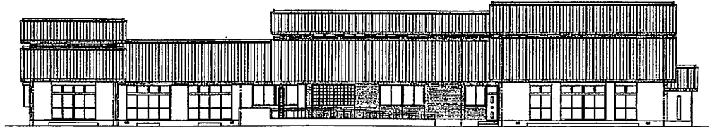
東側正面図
